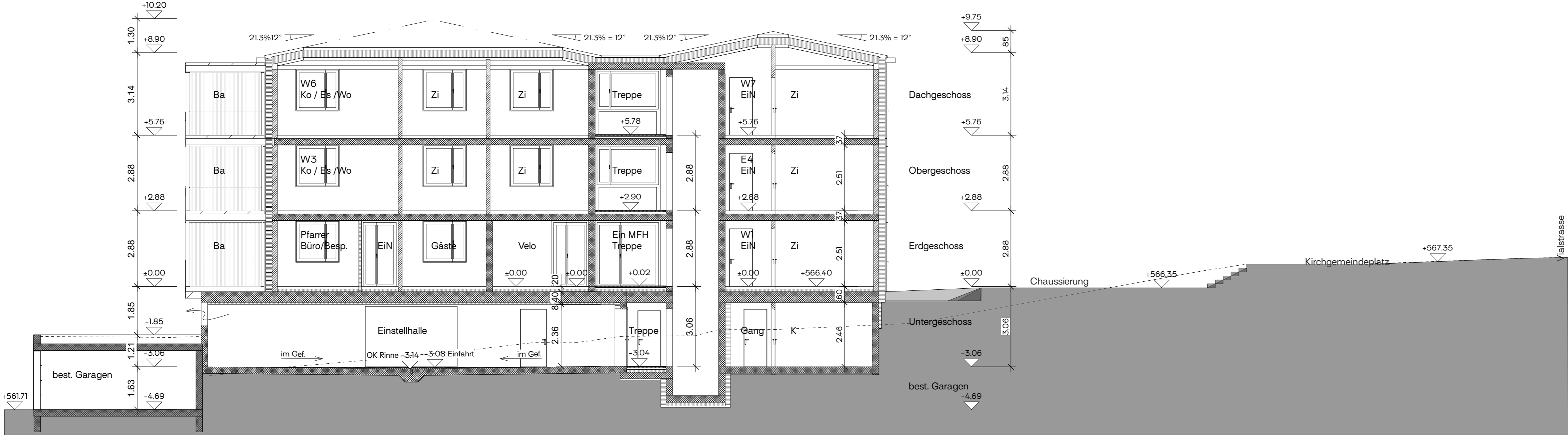
Schnitt C
