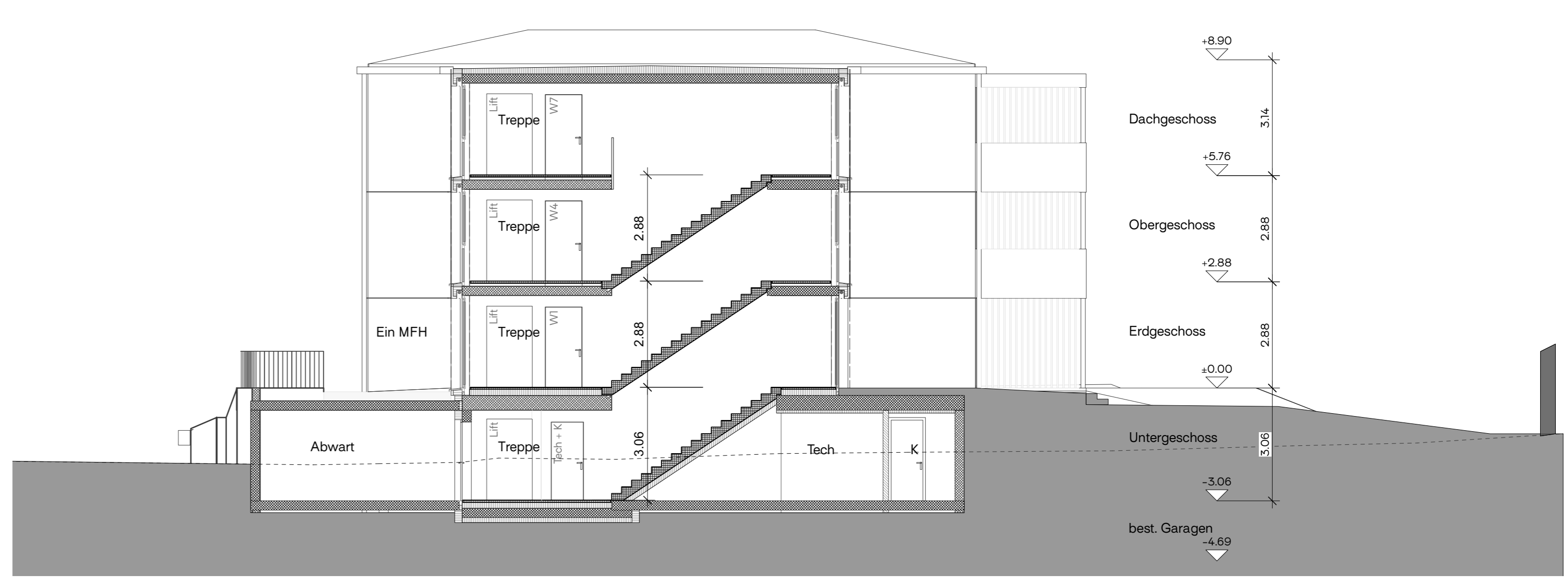
Schnitt B
