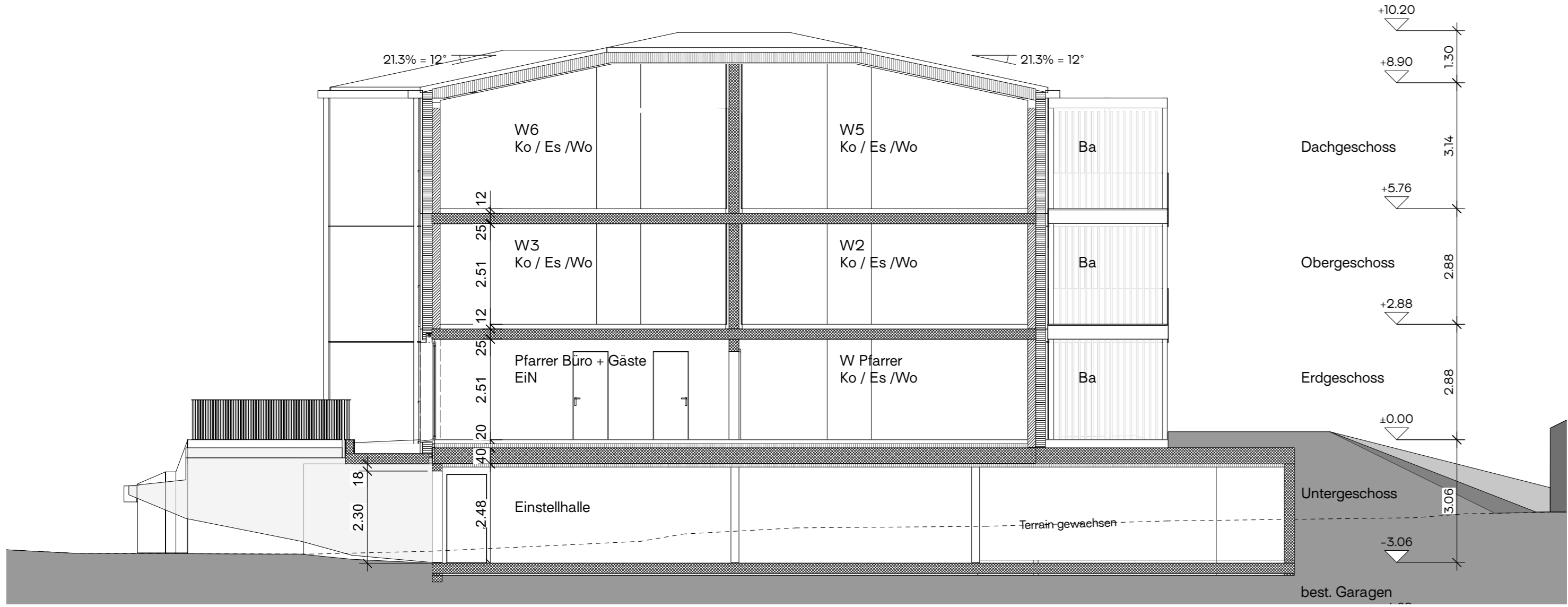
Schnitt A
